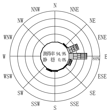
付図－A. 2. 77 高知西部沖 波高・波向別出現頻度図
