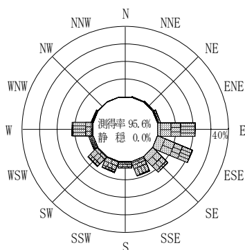
付図－A.2.71 静岡御前崎沖 波高・波向別出現頻度図
