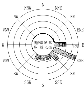
付図－A. 2. 73 三重尾鷲沖 波高・波向別出現頻度図
