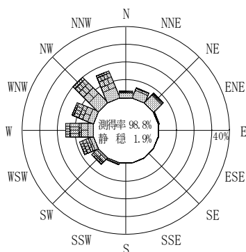
付図－A. 2. 61 青森西岸沖 波高・波向別出現頻度図
