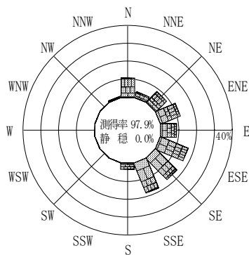
付図－A. 2. 65 岩手北部沖 波高・波向別出現頻度図
