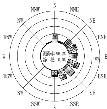
付図－A. 2. 66 岩手中部沖 波高・波向別出現頻度図
