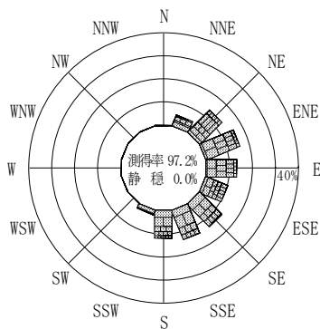
付図－A. 2. 68 宮城北部沖 波高・波向別出現頻度図
