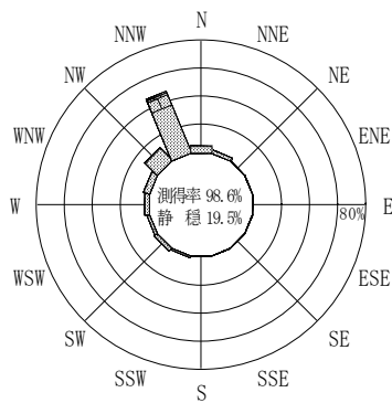
付図－A. 2. 59 平良沖 波高・波向別出現頻度図
