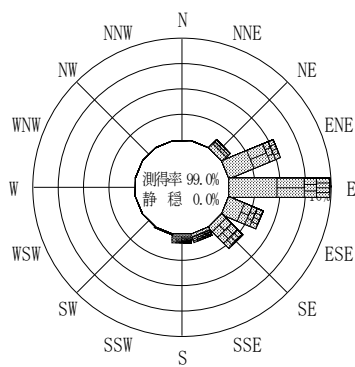
付図－A. 2. 58 中城湾 波高・波向別出現頻度図
