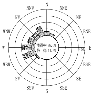
付図－A.2.1 留萌 波高・波向別出現頻度図
