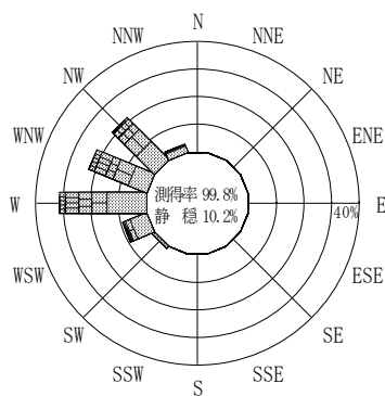
付図－A.2.3 瀬棚 波高・波向別出現頻度図
