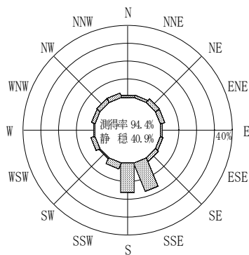
付図－A. 2. 47 伊勢湾 波高・波向別出現頻度図
