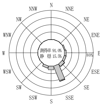
付図－A. 2. 45 清水 波高・波向別出現頻度図
