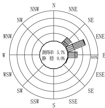
付図－A. 2. 55 細島 波高・波向別出現頻度図
