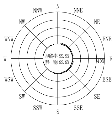
付図－A. 2. 57 鹿児島 波高・波向別出現頻度図
