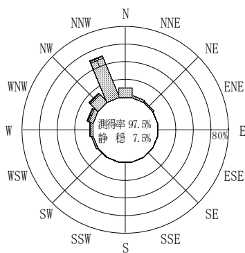
付図－A.2.21 藍島 波高・波向別出現頻度図
