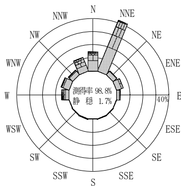
付図－A. 2. 22 玄界灘 波高・波向別出現頻度図
