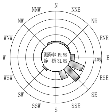
付図－A. 2. 50 小松島 波高・波向別出現頻度図
