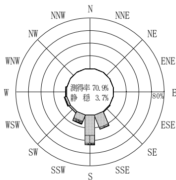
付図－A.2.51 室津 波高・波向別出現頻度図
