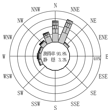
付図－A.2.20 浜田 波高・波向別出現頻度図
