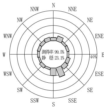
付図－A.2.42 第二海堡 波高・波向別出現頻度図
