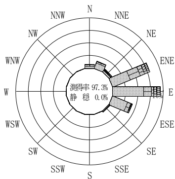
付図－A. 2. 32 八戸 波高・波向別出現頻度図
