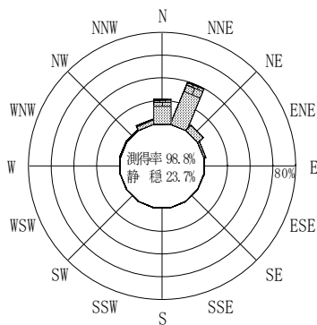
付図－A.2.10 富山 波高・波向別出現頻度図
