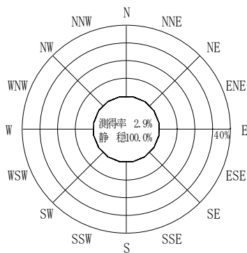
付図－A.2.12 輪島 波高・波向別出現頻度図
