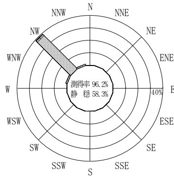
(f5 : 4.6~7.5秒) 2012年 1月~2012年12月
