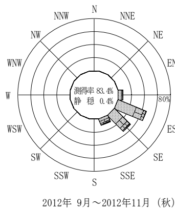
付図-B.2.37 仙台新港 波高・波向別出現頻度図（連続観測）
