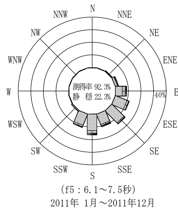
付図-B.3.72 三重尾鷲沖 波高・波向別出現頻度図 (連続観測, f2, f3, f4, f5, 全周期帯)
