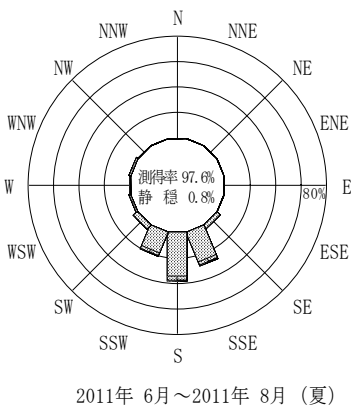
付図-B.2.43 アシカ島 波高・波向別出現頻度図（連続観測）
