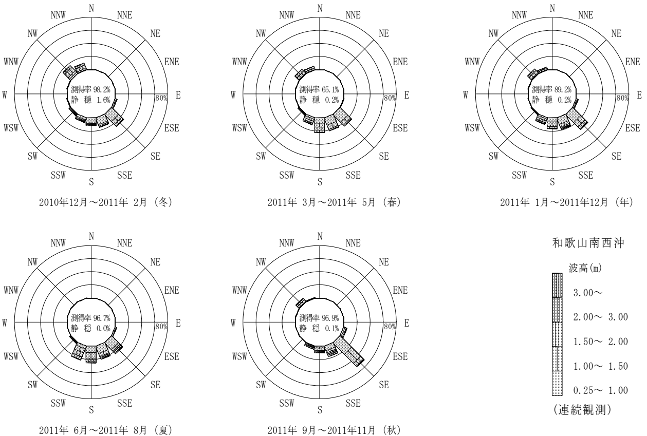
付図-B.2.73 和歌山南西沖 波高・波向別出現頻度図 (連続観測)
