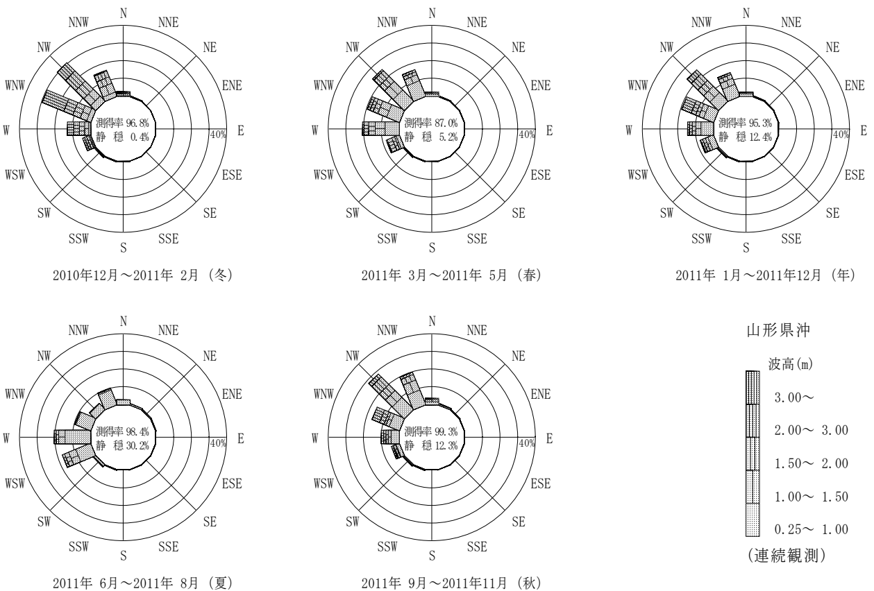
付図-B.2.63 山形県沖 波高・波向別出現頻度図（連続観測）
