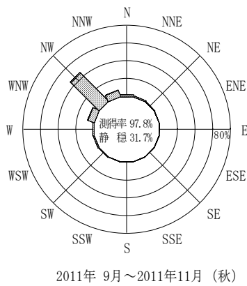
付図-B.2.60 石垣沖 波高・波向別出現頻度図(連続観測)
