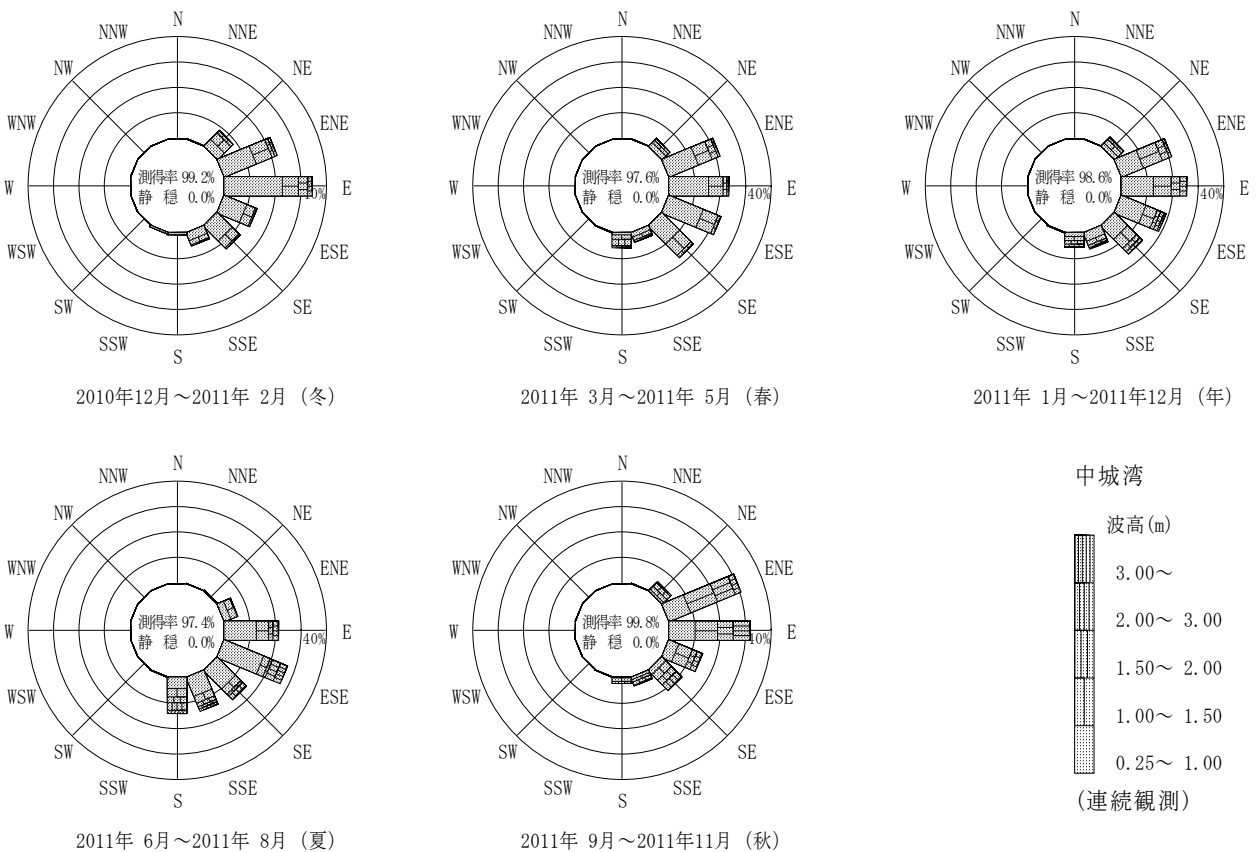
付図-B.2.58 中城湾 波高・波向別出現頻度図(連続観測)
