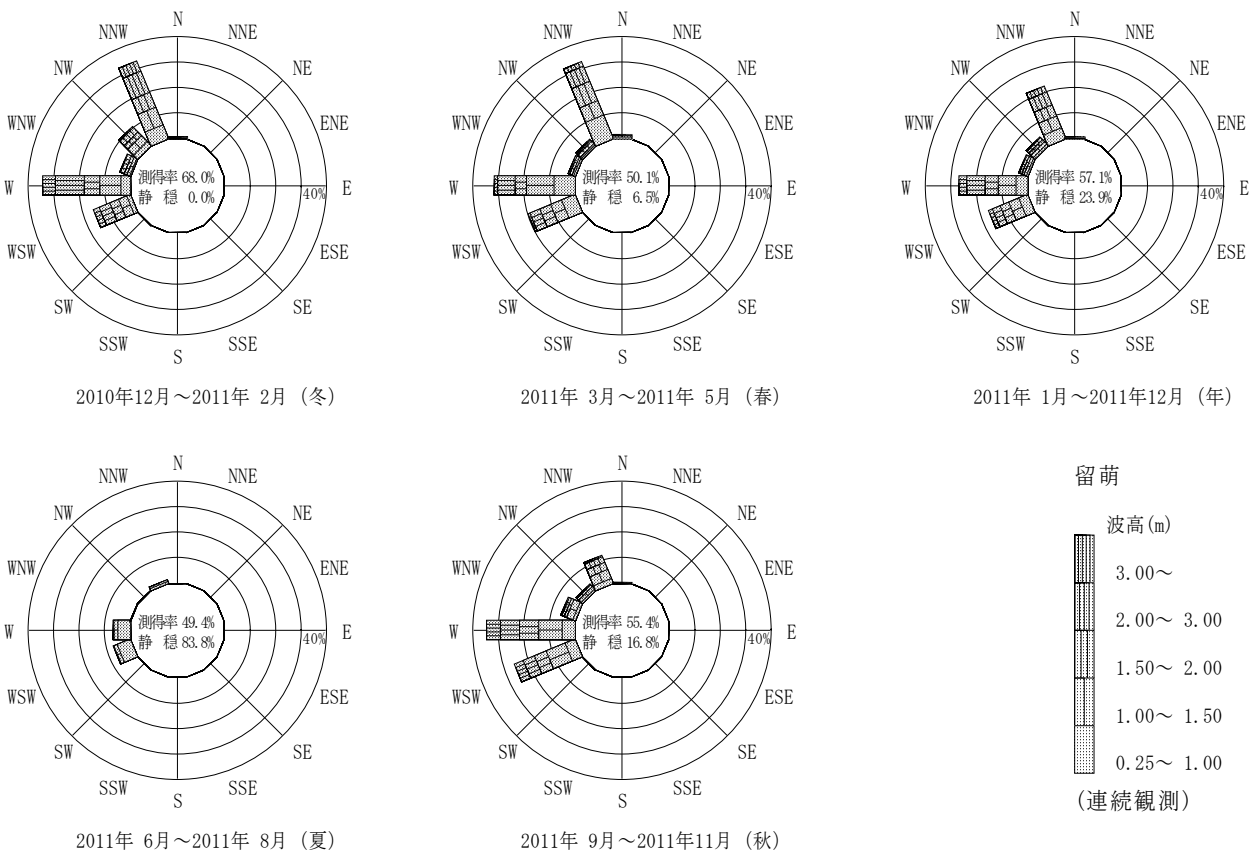
付図-B.2.1 留萌 波高・波向別出現頻度図（連続観測）
