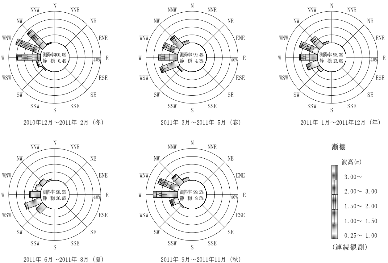
付図-B.2.3 瀬棚 波高・波向別出現頻度図（連続観測）
