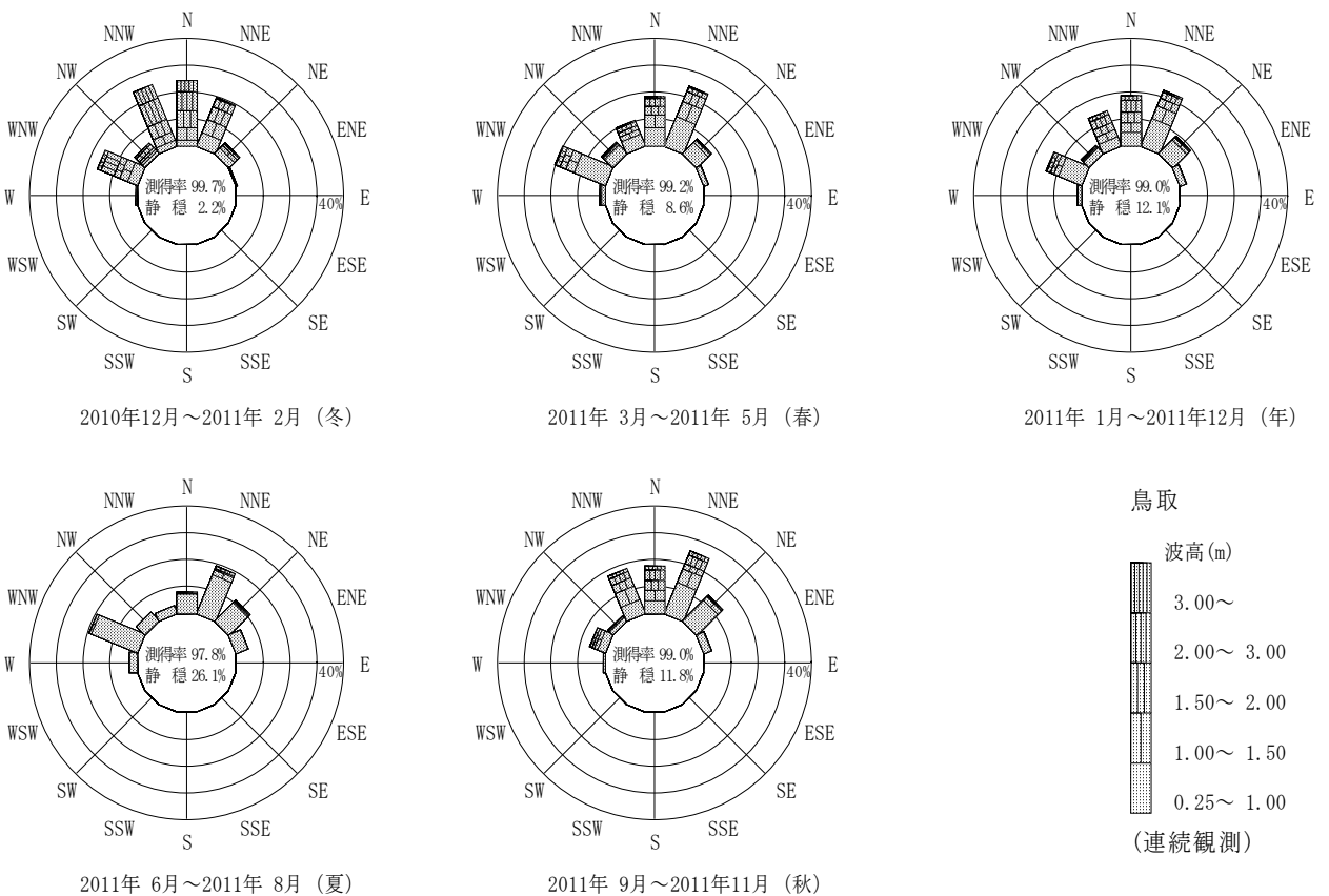
付図-B.2.18 鳥取 波高・波向別出現頻度図（連続観測）
