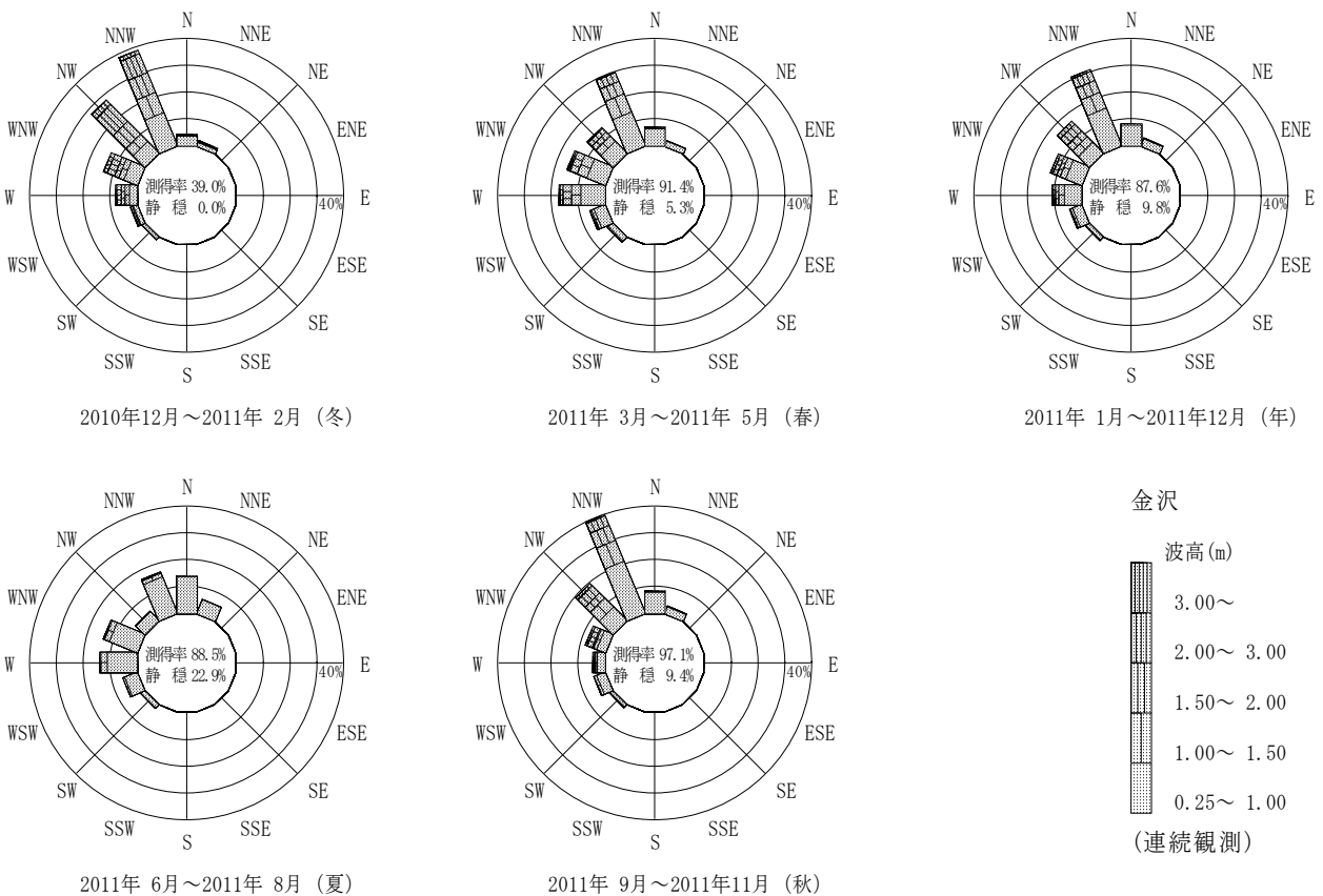
付図-B.2.13 金沢 波高・波向別出現頻度図（連続観測）
