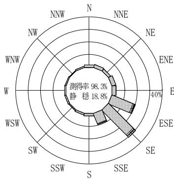
付図-A.2.50 小松島 波高・波向別出現頻度図
