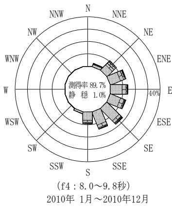
付図-B.3.66 宮城北部沖 波高・波向別出現頻度図 (連続観測, f2, f3, f4, f5, 全周期帯)
