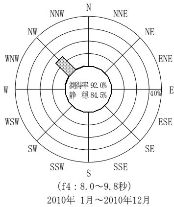
付図-B.3.61 石垣沖 波高・波向別出現頻度図(連続観測, f2, f3, f4, f5, 全周期帯)
