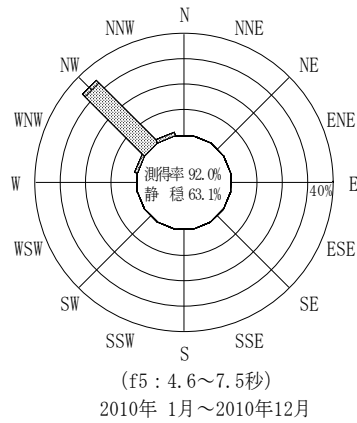
付図-B.3.61 石垣沖 波高・波向別出現頻度図(連続観測, f2, f3, f4, f5, 全周期帯)
