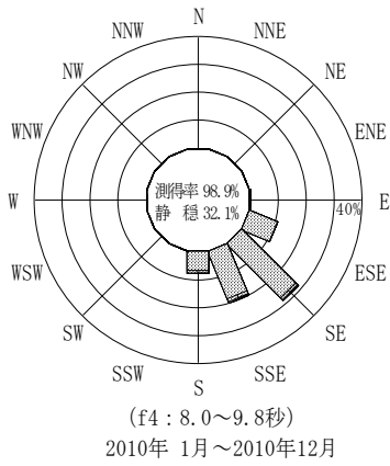
付図-B.3.47 御前崎 波高・波向別出現頻度図(連続観測, f2, f3, f4, f5, 全周期帯)
