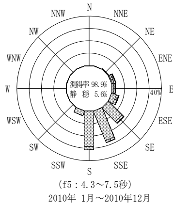
付図-B.3.47 御前崎 波高・波向別出現頻度図(連続観測, f2, f3, f4, f5, 全周期帯)
