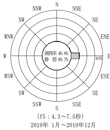
付図-B.3.55 苧田 波高・波向別出現頻度図 (連続観測, f2, f3, f4, f5, 全周期帯)
