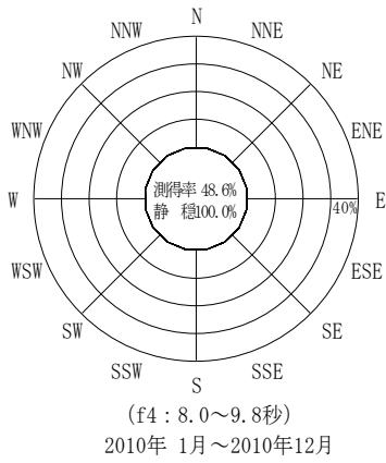
付図-B.3.55 苧田 波高・波向別出現頻度図 (連続観測, f2, f3, f4, f5, 全周期帯)
