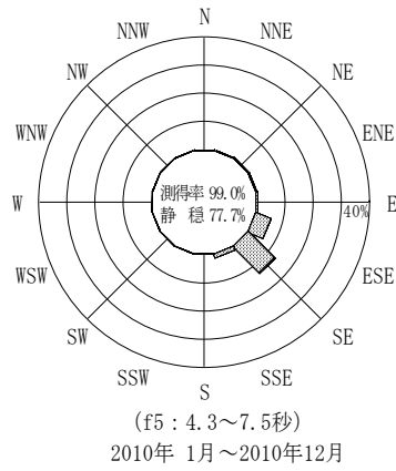
付図-B.3.51 小松島 波高・波向別出現頻度図(連続観測, f2, f3, f4, f5, 全周期帯)
