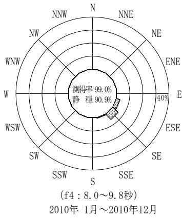
付図-B.3.51 小松島 波高・波向別出現頻度図(連続観測, f2, f3, f4, f5, 全周期帯)
