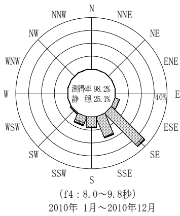
付図-A.3.71 和歌山南西沖 波高・波向別出現頻度図 (f2, f3, f4, f5, 全周期帯)
