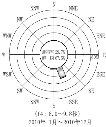
付図-A.3.46 清水 波高・波向別出現頻度図 (f2, f3, f4, f5, 全周期帯)
