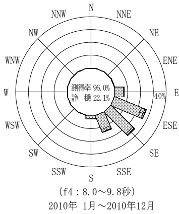
付図-A.3.56 細島 波高・波向別出現頻度図 (f2, f3, f4, f5, 全周期帯)
