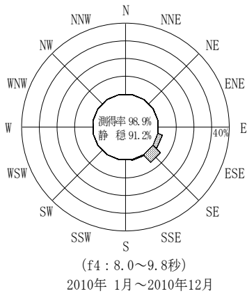
付図-A.3.51 小松島 波高・波向別出現頻度図 (f2, f3, f4, f5, 全周期帯)
