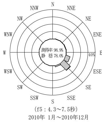
付図-A.3.51 小松島 波高・波向別出現頻度図 (f2, f3, f4, f5, 全周期帯)
