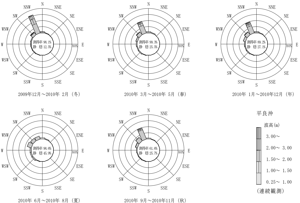
付図-B.2.60 平良沖 波高・波向別出現頻度図(连续観測)
