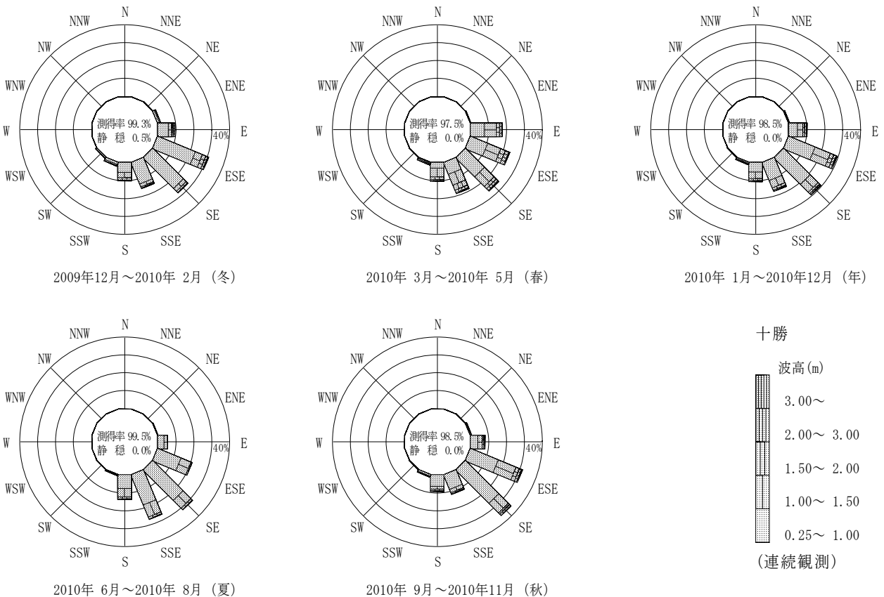
付図-B.2.29 十勝 波高・波向別出現頻度図(連続観測)
