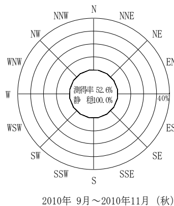
付図-B.2.48 伊勢湾 波高・波向別出現頻度図(連続観測)
