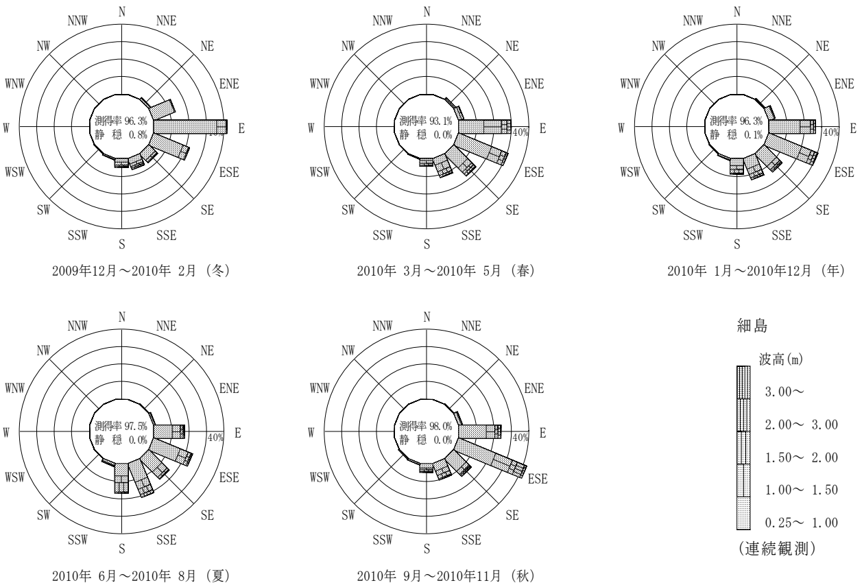
付図-B.2.56 細島 波高・波向別出現頻度図（連続観測）
